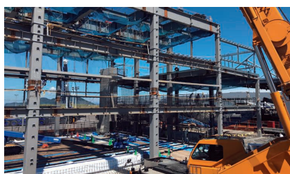
建設中のパワートレイン試験棟
