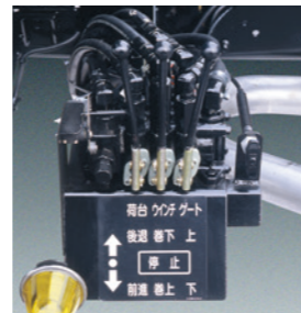
手動操作レバー
