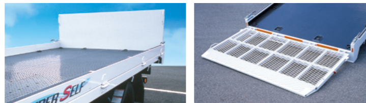
125mm開閉式横アオリと700mm全面縞鋼板張道板 1,150mm全面エキスパンドメタル張道板
